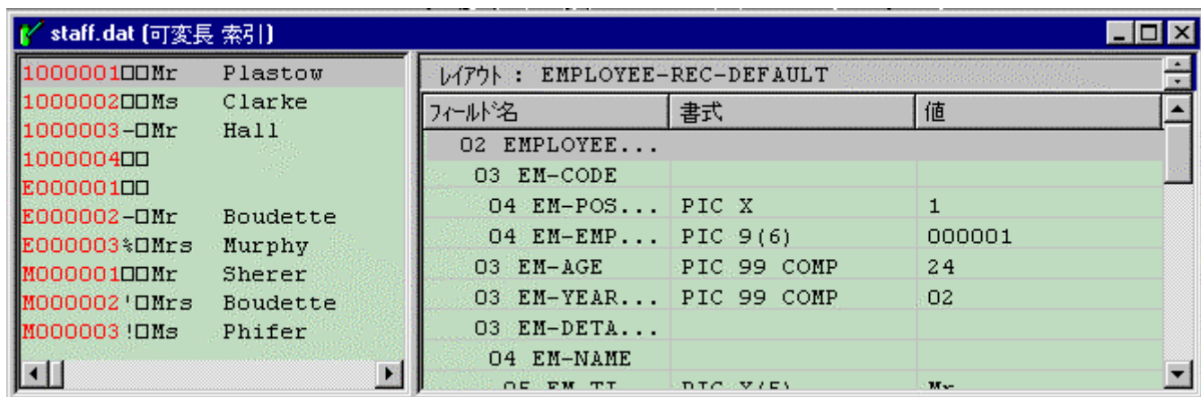
図 11-1: 「データファイルエディタ」ウィンドウ
