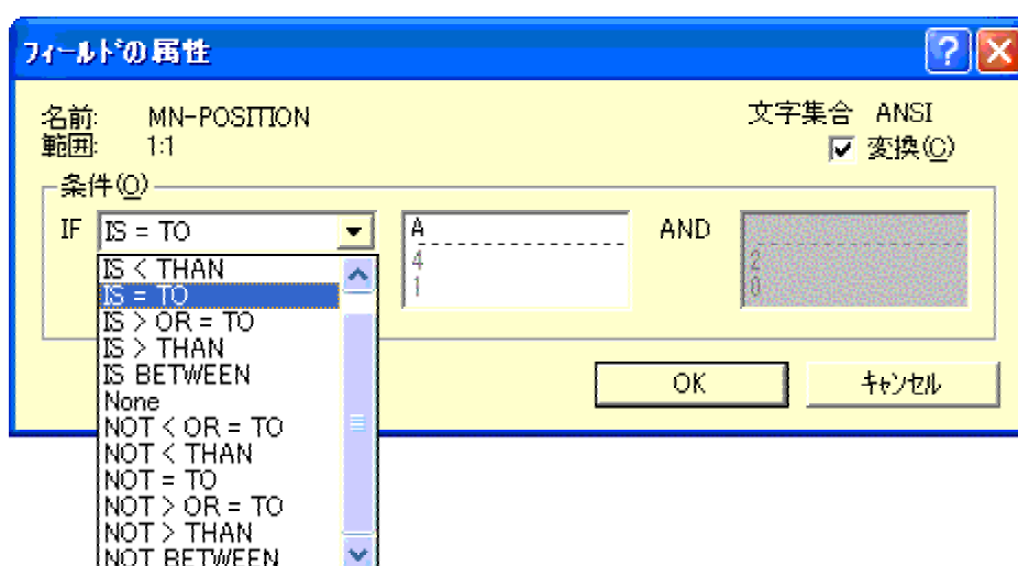
図 12-6: 「フィールドの属性」ダイアログボックスでの条件の指定
