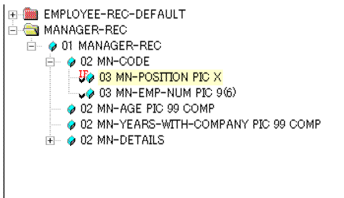
図 12-5: レコードレイアウトビュー
