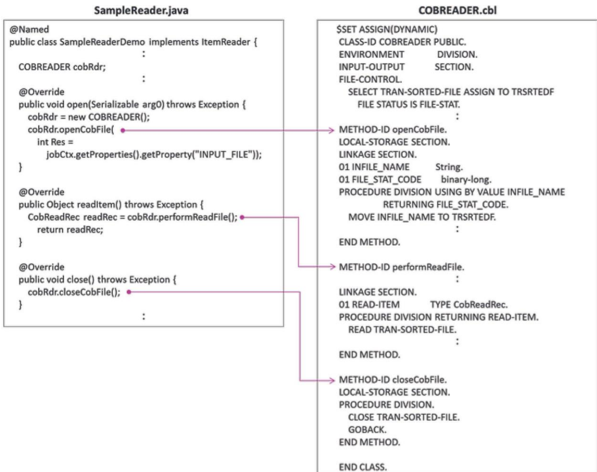
図 6 - 5 Reader による COBOL データファイルアクセスロジック例
