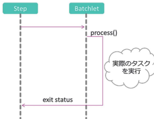
図 5-2 Batchlet Step の処理フロー
