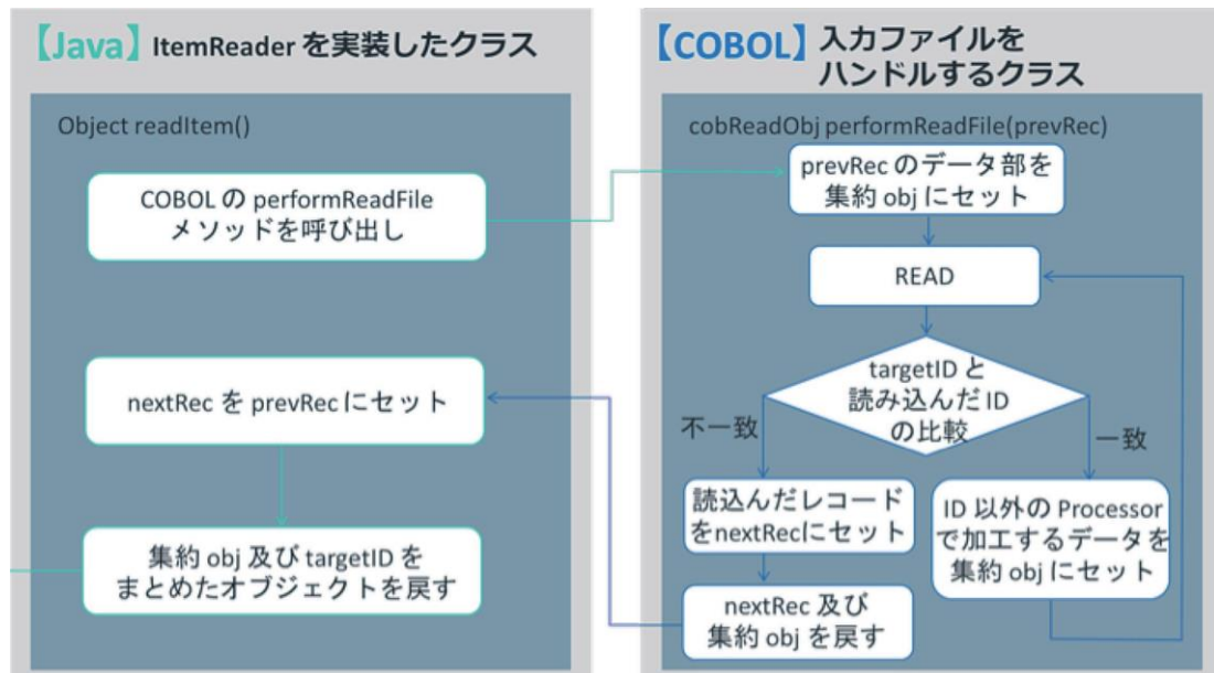
図6- 7 入力レコードの集約化の例
