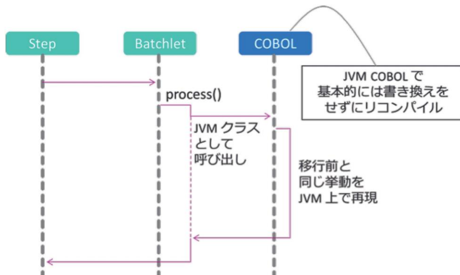
図 6- 1 Batchlet ステップ内で COBOL 資産を利用
